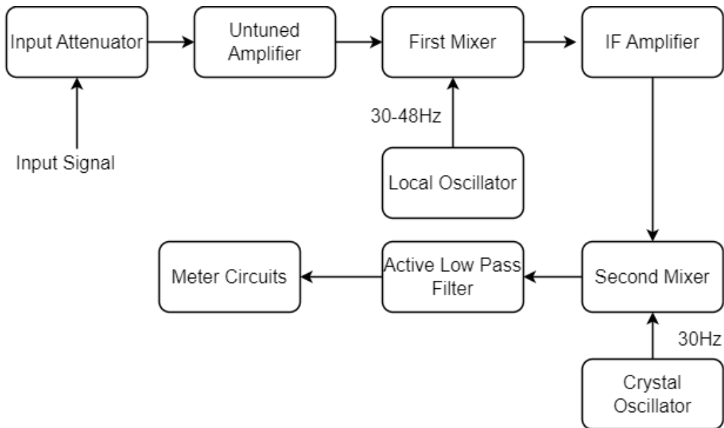
Fig: Heterodyne Wave Analyzer
